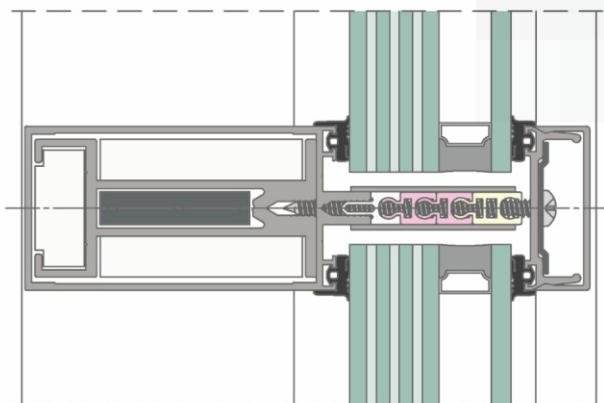
PRZEKRÓJ PRZEZ RYGIEL
