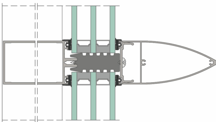
PRZEKRÓJ PRZEZ RYGIEL
