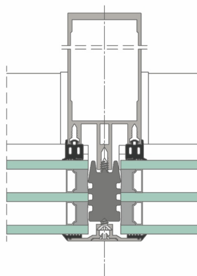
PRZEKRÓJ PRZEZ SŁUP
