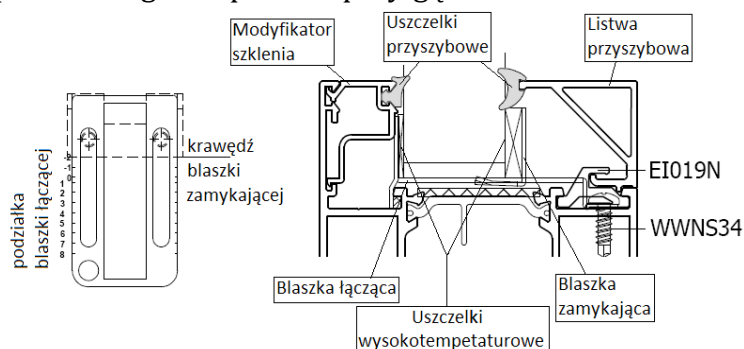
Rysunek nr 8: Przykładowy schemat mocowania i uszczelnienia wypełnienia przeziernego / nieprzeziernego dla profili z przylgą na szklenie
