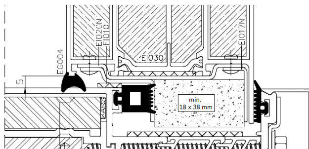
Rysunek nr 14: Przykładowy schemat mocowania i uszczelnienia w ścianie osłonowej PONZIO PF 152
