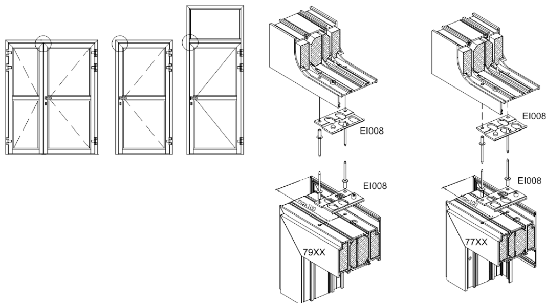
Rysunek nr 11: Montaż blokady dylatacyjnej
