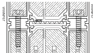
Rysunek nr 2: Łączenie profili dodatkowych ościeżnicy
