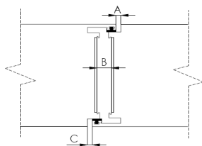
Rysunek nr 15: Oznaczenia szczelin pomiędzy skrzydłem a obwiednią skrzydła
