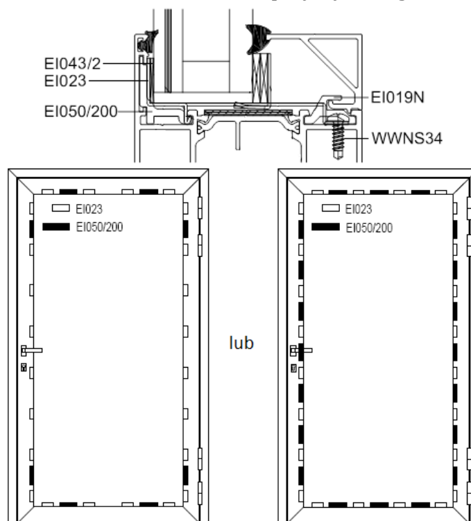
Rysunek nr 9: Schemat mocowania wzmocnienia przyszybowego
