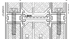
Rysunek nr 16: Łączenie profili dodatkowych ościeżnicy
