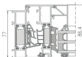
PRZEKRÓJ PRZES OKNO TM 77N HI+
