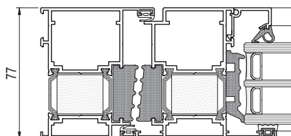
PRZEKRÓJ PRZESZ DRZWI TM 77N HI+ OTWIERANE NA ZEWNĄTRZ
